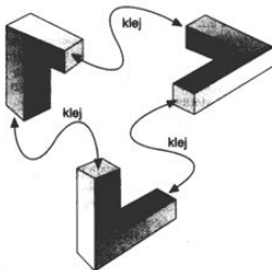
Rys. 3.21. Niemożliwy trójkąt. Nie można zlokalizować przyczyny niemożliwości, a mimo to da się ją ściśle zdefiniować matematycznie, analizując reguły sklejanía fragmentów.
