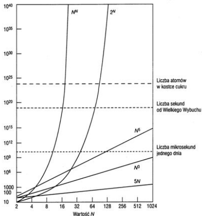
rys. 4.8 Tempo wzrostu wartości 5N , N^3 , N^5 i 2^N , wraz ze wzrostem N , w porównaniu z innymi wielkimi liczbami.
